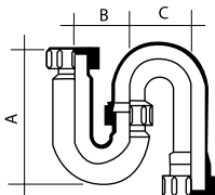
Tubular 'S' Trap
