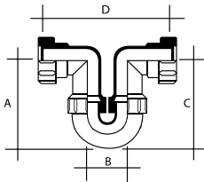
Tubular 'Running'
