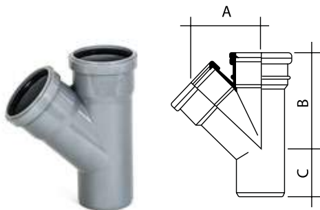
Y Branch 45°
